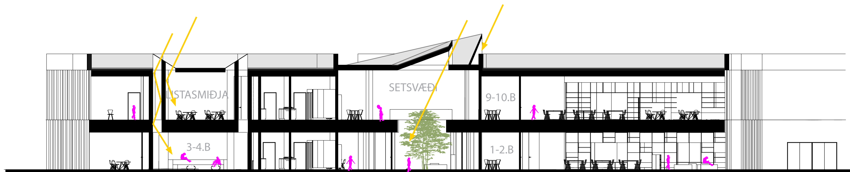
Þversnið
