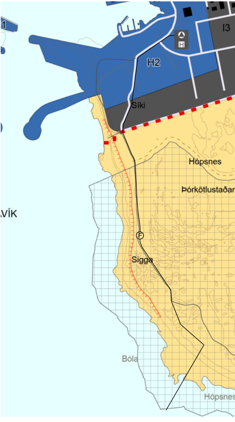
BREYTTUR AÐALSKIPULAGSUPPDRAÐTÚR 1:10.000 HREINSIVIRKI OG FRÁRENNSLI
