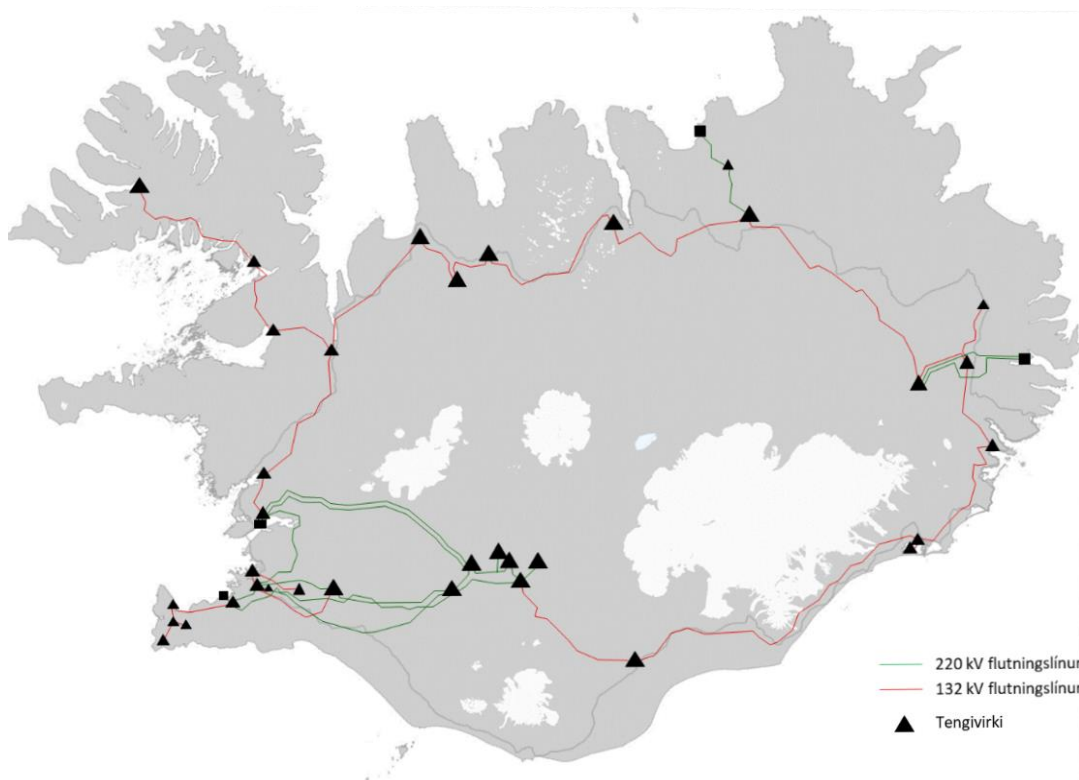
Mynd 2.1 Meginflutningskerfið 2019
