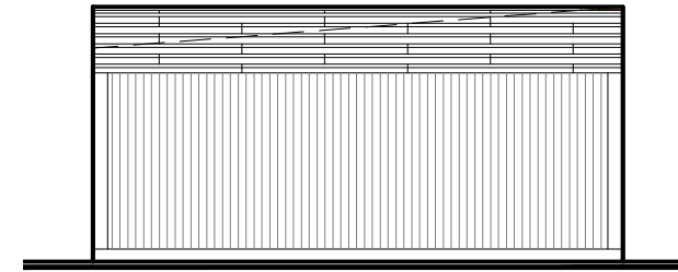
Bílskúr útlit Austur M= 1:100
