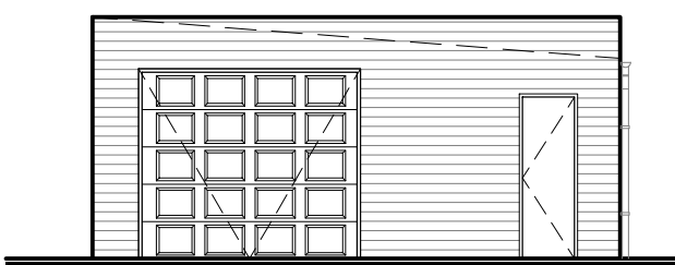
Bílskúr útlit Vestur M= 1:100
