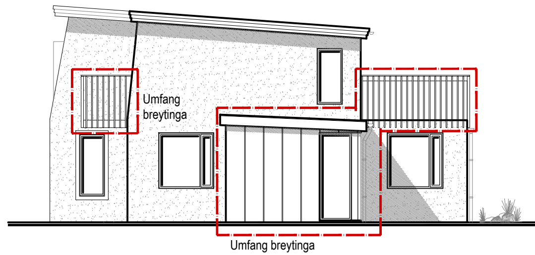
Útlit Suður M= 1:100
