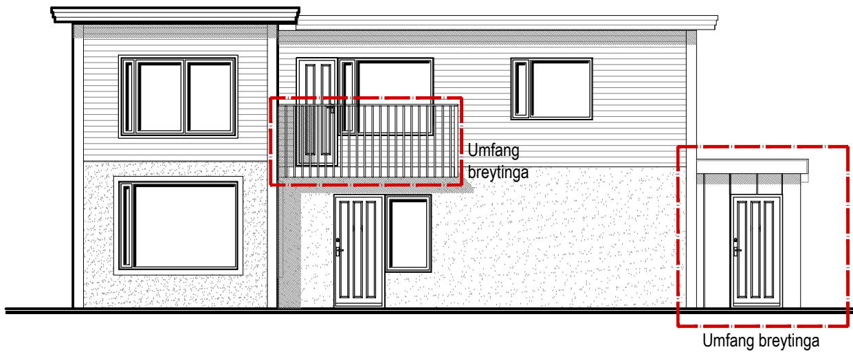
Útlit Vestur M= 1:100
