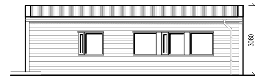
Bílskúr útlit Suður M= 1:100
