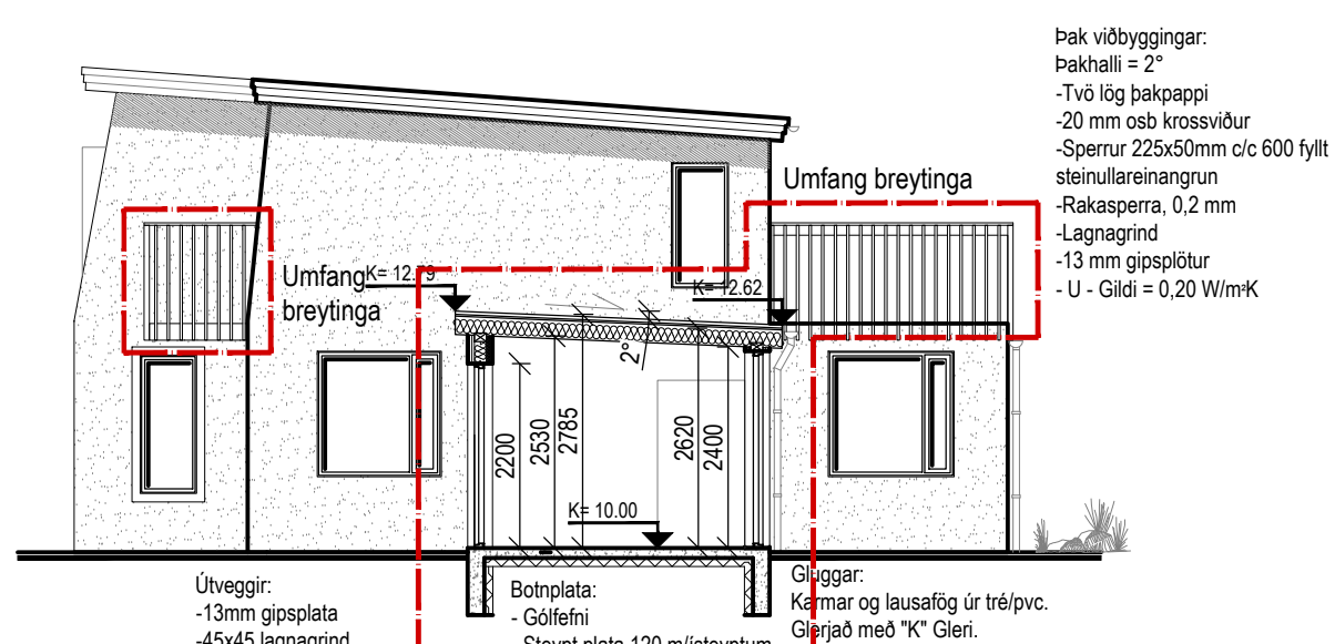
Snið B-B M= 1:100
