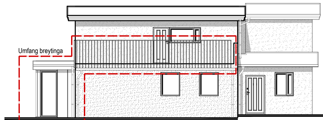
Útlit Austur M= 1:100
