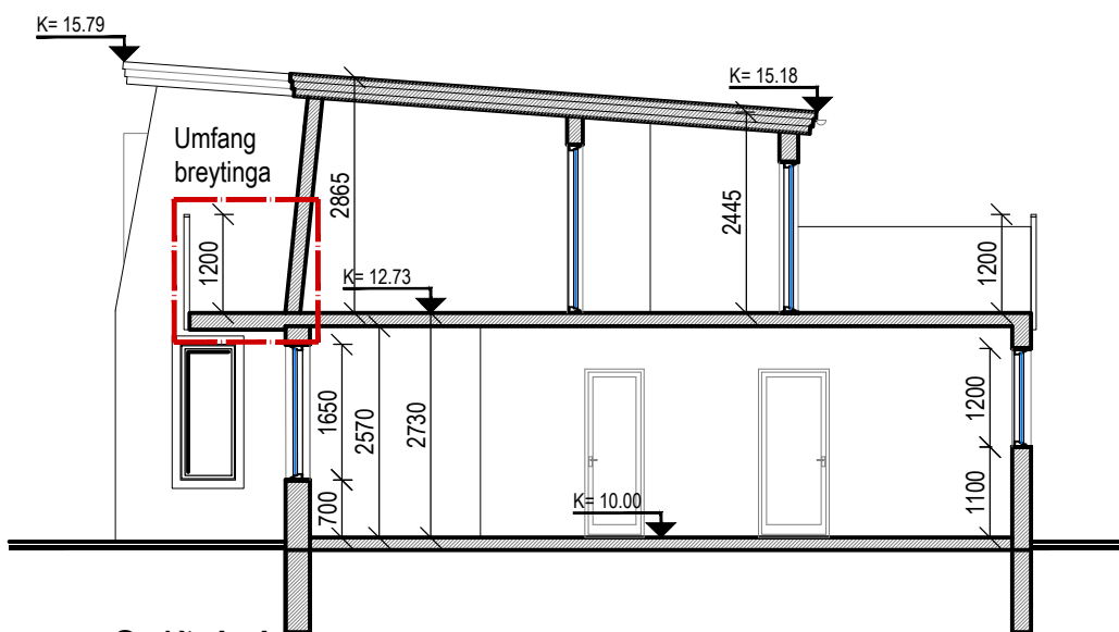
Snið A-A M= 1:100
